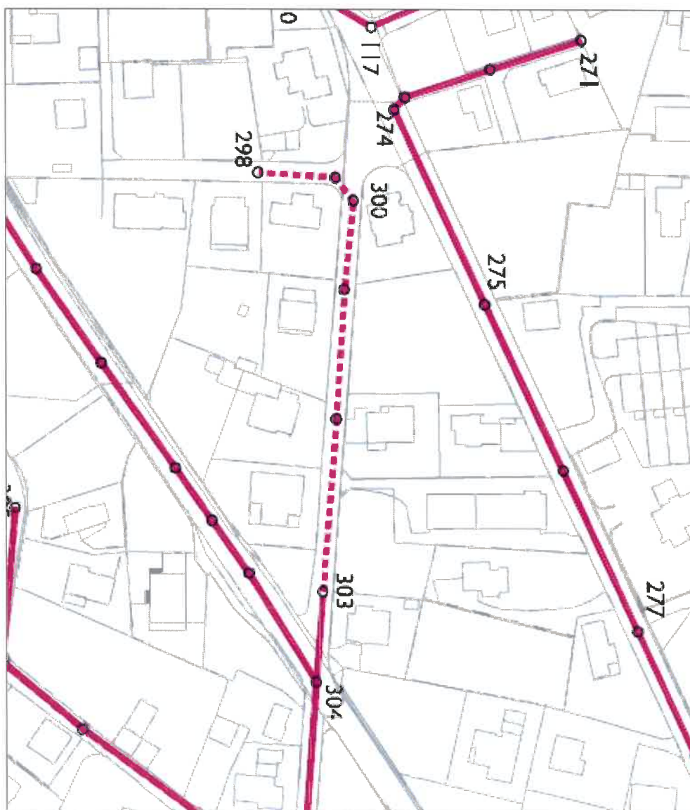
Planimetria intervento PGS (la condotta tratteggiata è da posare)
